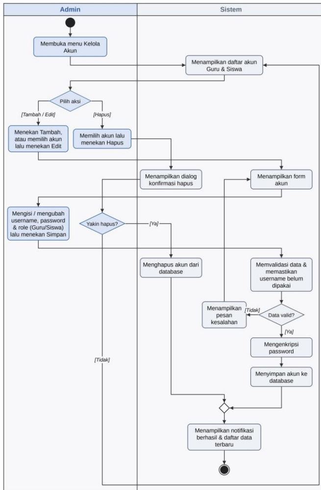
Gambar 2. Activity Diagram Kelola Akun Guru & Siswa
