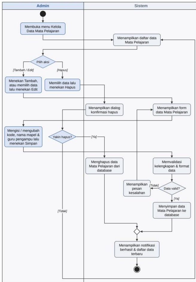
Gambar 6. Activity Diagram Kelola Data Mata Pelajaran
