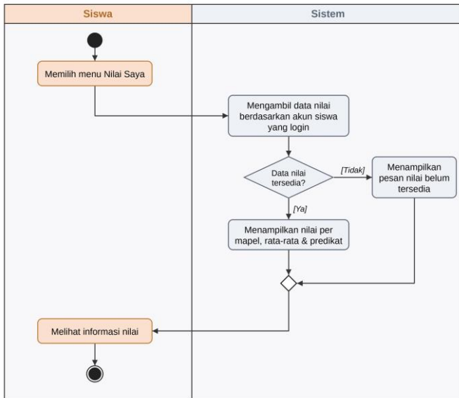
Gambar 11. Activity Diagram Lihat Nilai Sendiri (Siswa)
