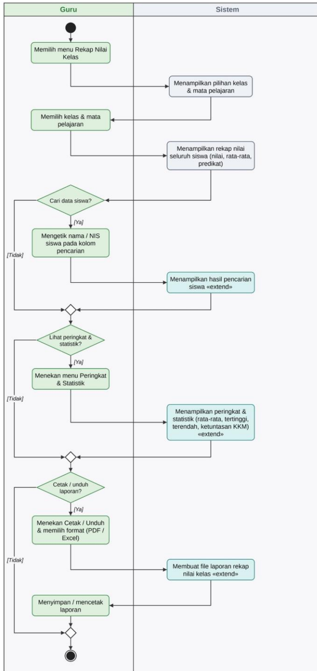
Gambar 10. Activity Diagram Lihat Rekap Nilai Kelas
